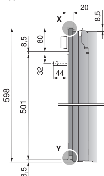
Appareil dans armoire haute
