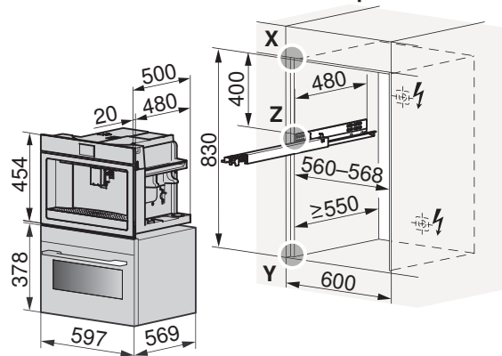
CoffeeCenter V6000 45 et four à vapeur
