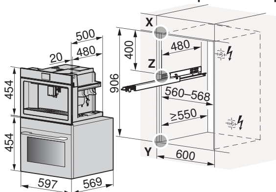
CoffeeCenter V6000 45 et four compact/four à vapeur
