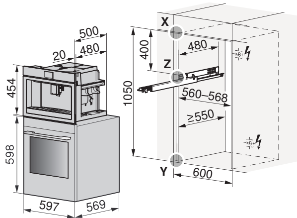
CoffeeCenter V6000 45 et four
