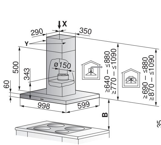
Plan de perçage (vue X)
