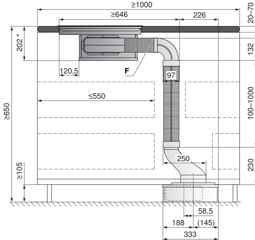
Montage îlot avec profondeur \geq 1000
