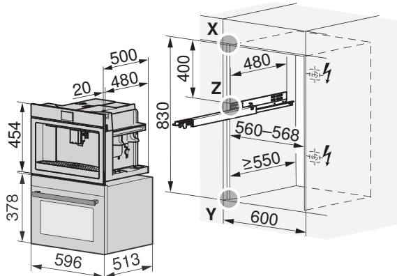
Dimensions de la façade des appareils: détail X/Y/Z (voir page 12)
